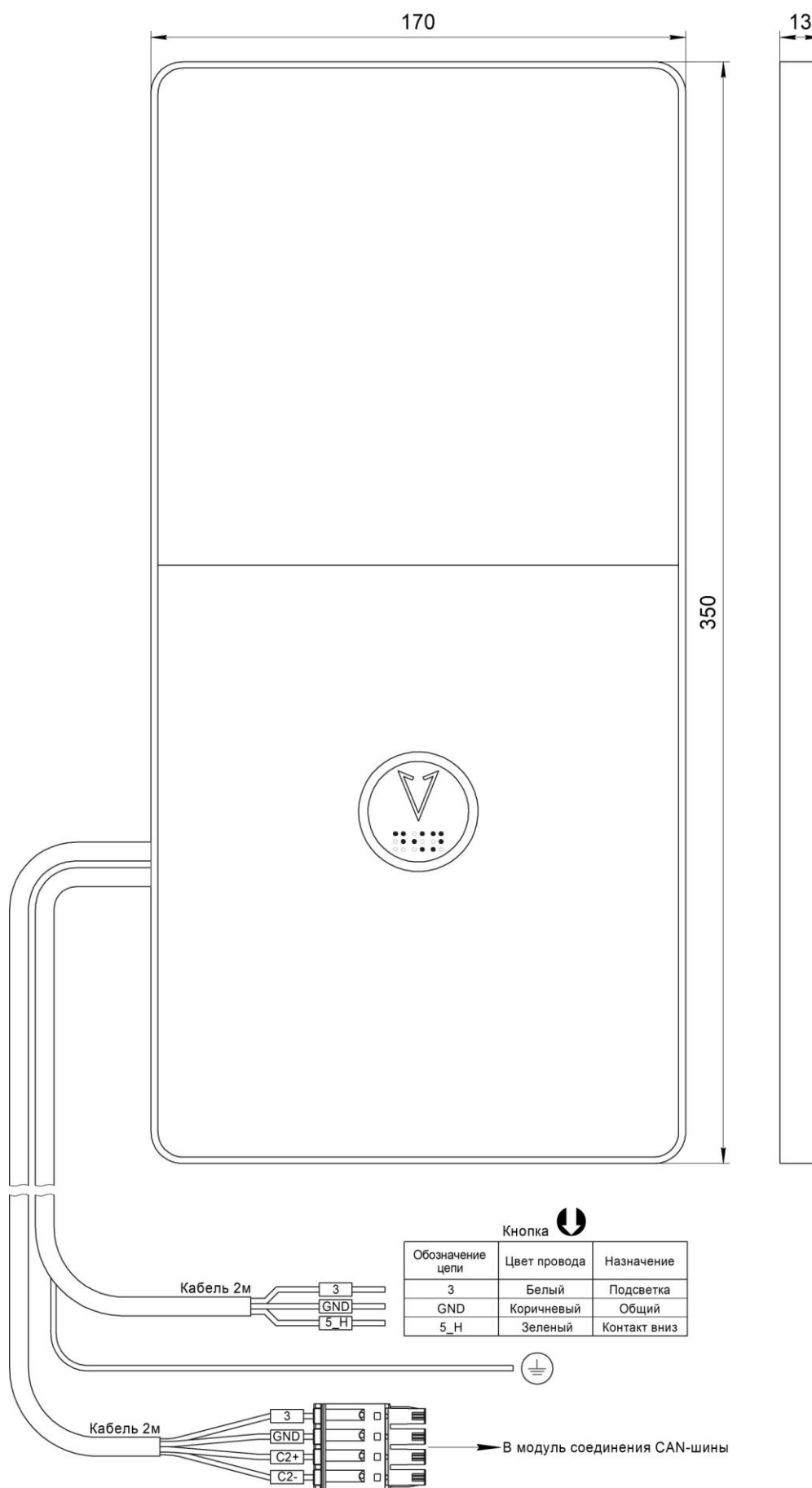
Рис.1 Внешний вид, габаритные и установочные размеры Вызывного поста МАЛАХИТ НШЕК.468381.017-01
